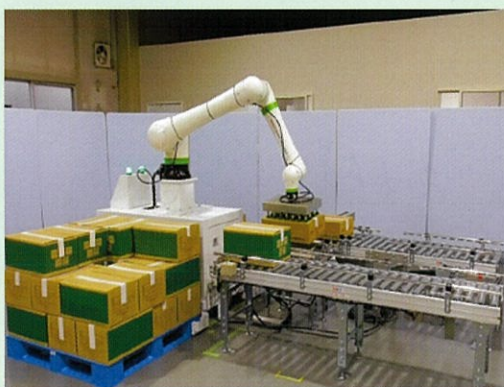
パレタイザ
