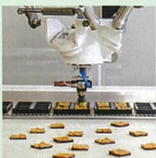
パッキング
